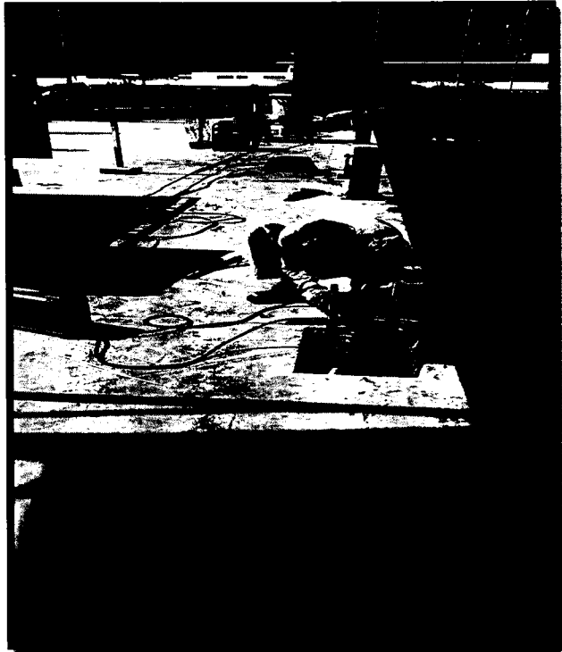
SOLDANDO EL FIERRO 5/8 Y 3/8" CON LA ESTRUCTURA EXISTENTE : VIGAS DE MUELLE
